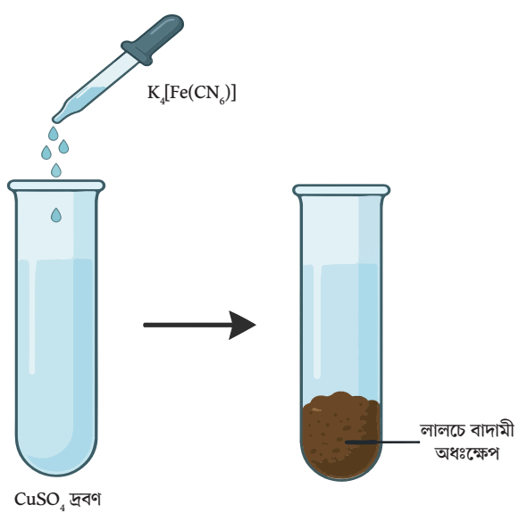
চিত্রঃ \text{K}_4[\text{Fe}(\text{CN})_6] দ্বারা \text{Cu}^{2+} আয়ন শনাক্তকরণ
