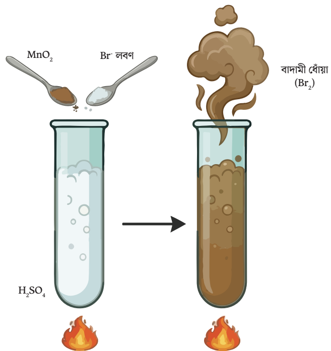
চিত্রঃ \text{Br}^- মূলকের সিন্ত পরিক্ষা
