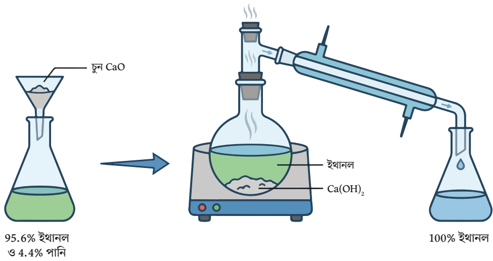
চিত্রঃ ইথানলের পাথুরে চুনসহ পাতন প্রক্রিয়ার নকশাচিত্র
