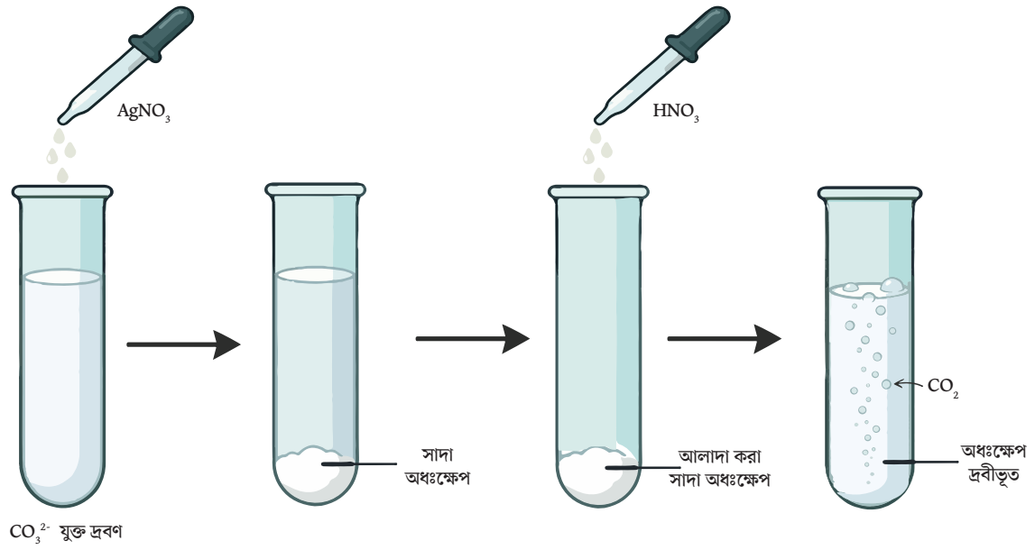
চিত্রঃ \text{AgNO}_3 দ্বারা \text{CO}_3^{2-} আয়ন শনাক্তকরণ
