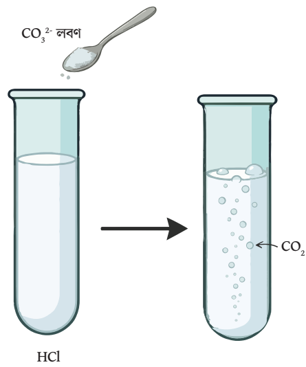
চিত্রঃ \text{CO}_3^{2-} মূলকের সিন্ত পরিক্ষা
