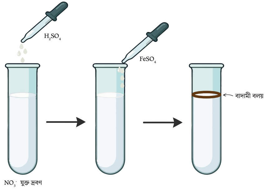
চিত্রঃ \text{NO}_3^- আয়ন শনাক্তকরণের বলয় পরিক্ষা
