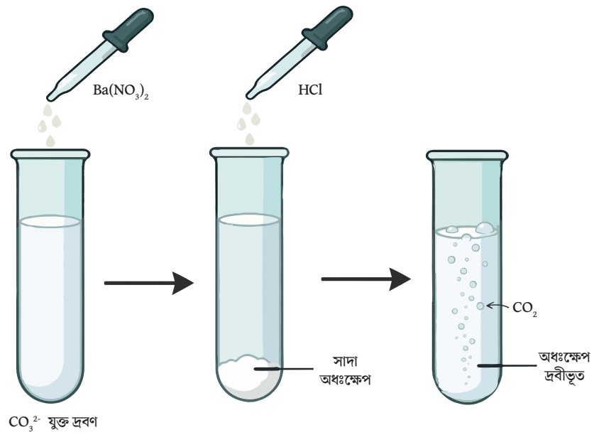
চিত্রঃ \text{Ba}(\text{NO}_3)_2 দ্বারা \text{CO}_3^{2-} আয়ন শনাক্তকরণ
