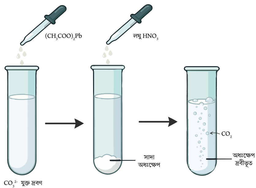
চিত্রঃ (\text{CH}_3\text{COO})_2\text{Pb} দ্বারা \text{CO}_3^{2-} আয়ন শনাক্তকরণ
