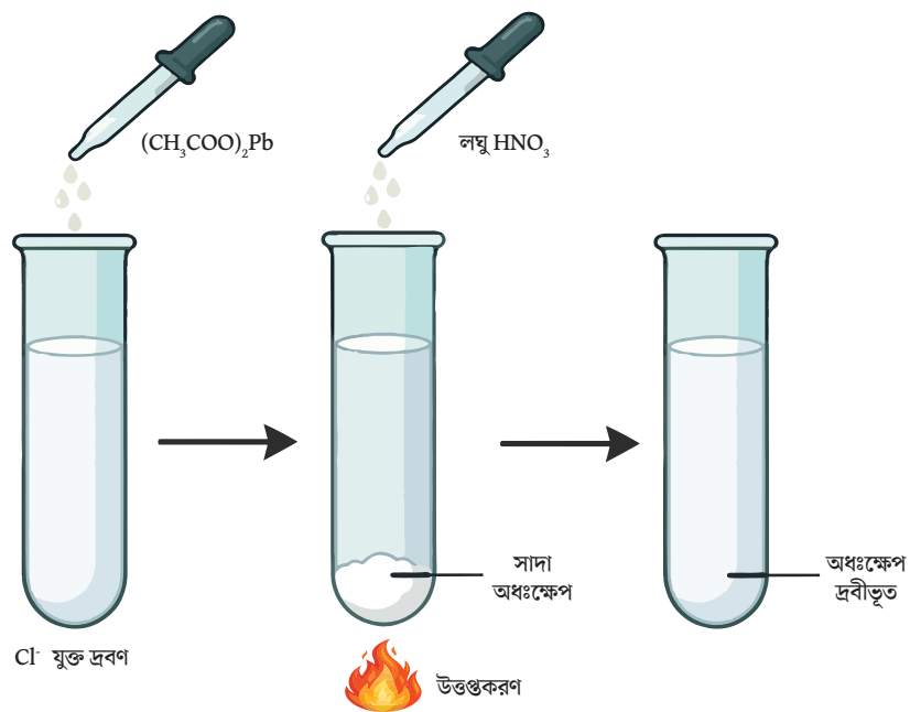
চিত্রঃ (\text{CH}_3\text{COO})_2\text{Pb} দ্বারা \text{Cl}^- আয়ন শনাক্তকরণ
