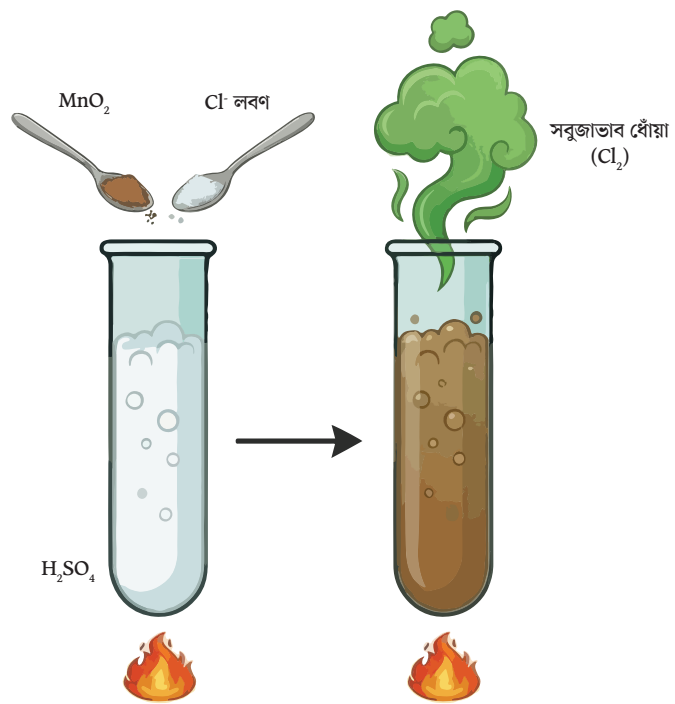
চিত্রঃ \text{Cl}^- মূলকের সিন্ত পরিক্ষা
