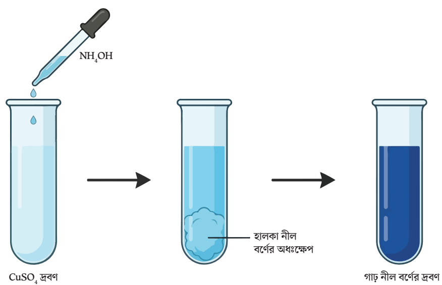
চিত্রঃ \text{NH}_4\text{OH} দ্বারা \text{Cu}^{2+} আয়ন শনাক্তকরণ
