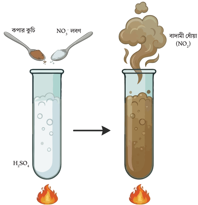
চিত্রঃ \text{NO}_3^- মূলকের সিন্ত পরিক্ষা
