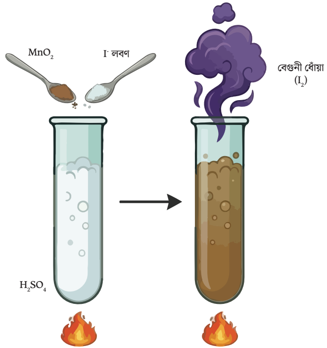
চিত্রঃ \text{I}^- মূলকের সিন্ত পরিক্ষা
