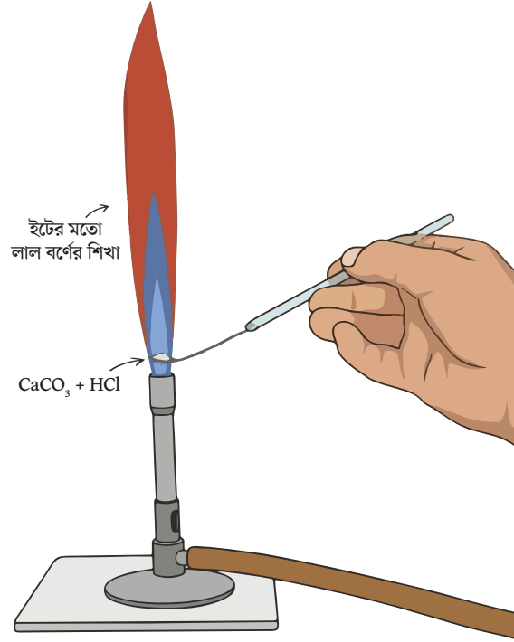
চিত্রঃ \text{CaCO}_3 এর শিখা পরিক্ষায় উৎপন্ন ইটের মতো লাল বর্ণের শিখা
