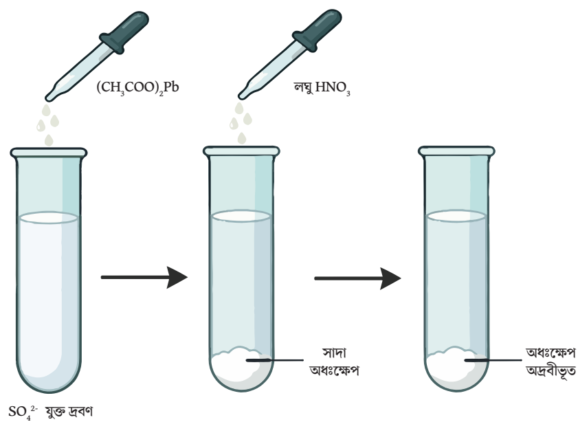
চিত্রঃ (\text{CH}_3\text{COO})_2\text{Pb} দ্বারা \text{SO}_4^{2-} আয়ন শনাক্তকরণ
