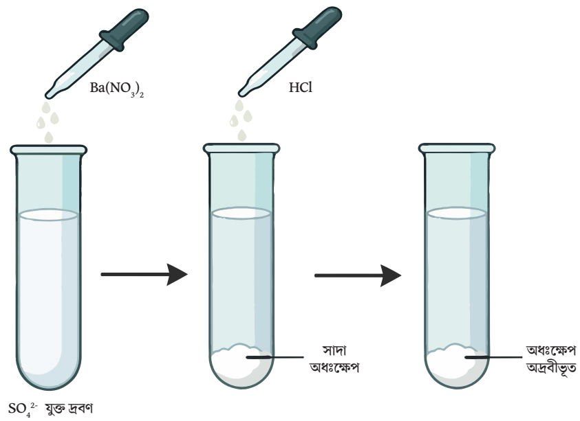
চিত্রঃ \text{Ba}(\text{NO}_3)_2 দ্বারা \text{SO}_4^{2-} আয়ন শনাক্তকরণ
